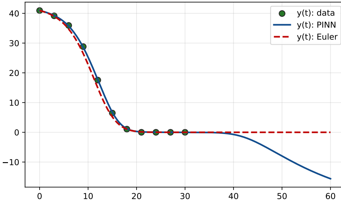
y(t): Fructose
