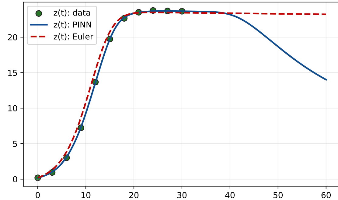
z(t): Ethanol
